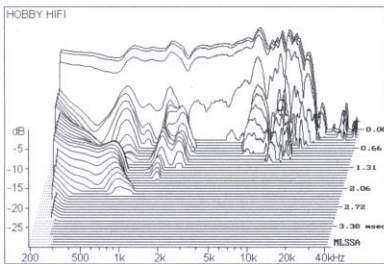
Leichte Resonanzanfälligkeit in den Mitteln.
