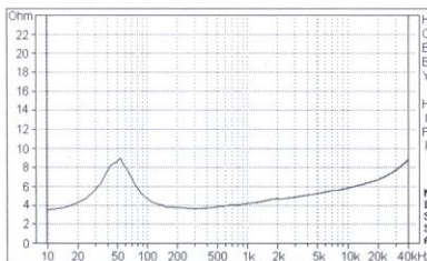
Sehr niedrige Schwingspuleninduktivität, stark bedämpfte Resonanzspitze.
