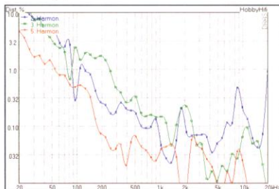
Unter 200 Hz relativ hoher Klirr, im Mittelhochtonbereich sehr geringe Verzerrungen.
