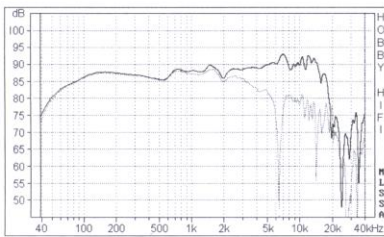
Nicht perfekt linear, aber wunderbar ausgewogen bis 15 kHz.
